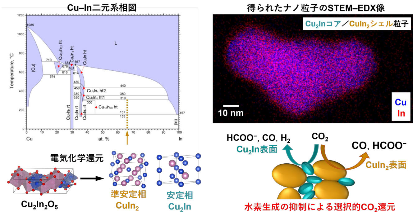
図 1. 電気化学的な非平衡構造再編成を利用した準安定な金属間化合物 CuIn 2 を含むナノ粒子の合成。相図は、物質・材料研究機構 (NIMS) のデータ中核拠点が提供する MatNavi から、Okamoto, H.; Massalski, T. Binary Alloy Phase Diagrams; ASM 617 International: 1990; Vol. 12, pp 3528–3531. に記載のデータを用いた図を引用。
