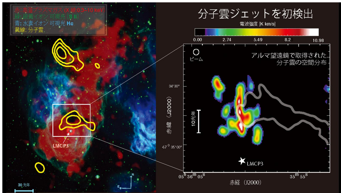
図 1. 大マゼラン雲のガンマ線連星系 LMC P3 周辺で発見された分子雲ジェット (左)大マゼラン雲の超新星残骸 DEM L241 と高エネルギー連星 LMC P3。赤は X 線、 緑・青は可視光、黄線は分子ガスを示す。(右)白枠内をアルマ望遠鏡で拡大した画像。色は分 子ガスの電波強度を表す。
