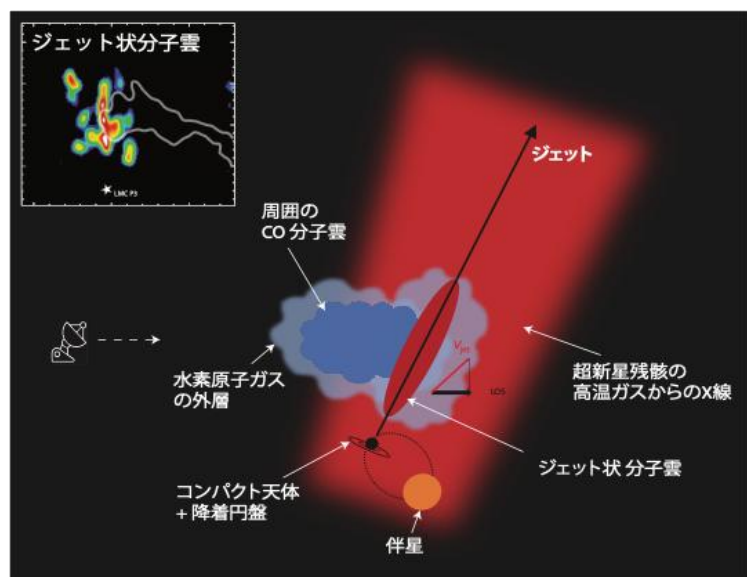
図 2. 高エネルギージェットによる相互作用の模式図 LMC P3のジェットが周囲の分子ガスと衝突し、細長い分子雲を形成した可能性を示す模式図。
