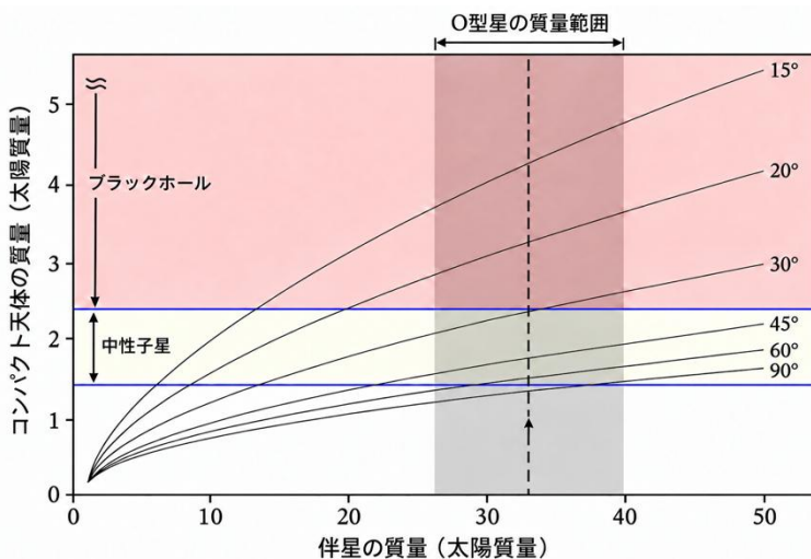
図 3: LMC P3 の伴星質量と軌道傾斜角から推定されるコンパクト天体の質量 (van Soelen et al. 2019) を改変。
