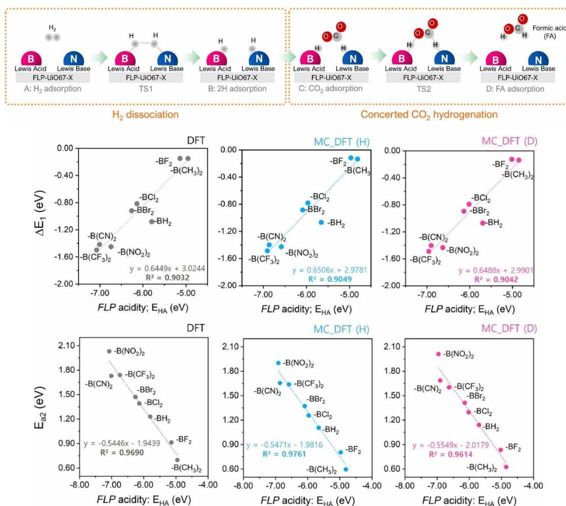
図1 FLP酸性度指標であるヒドリド付加エネルギー( E_{\text{HA}} )と、 \text{H}_2 解離の反応エネルギー( \Delta E_1 )および \text{CO}_2 水素化反応の活性化エネルギー( E_{a2} )との相関
