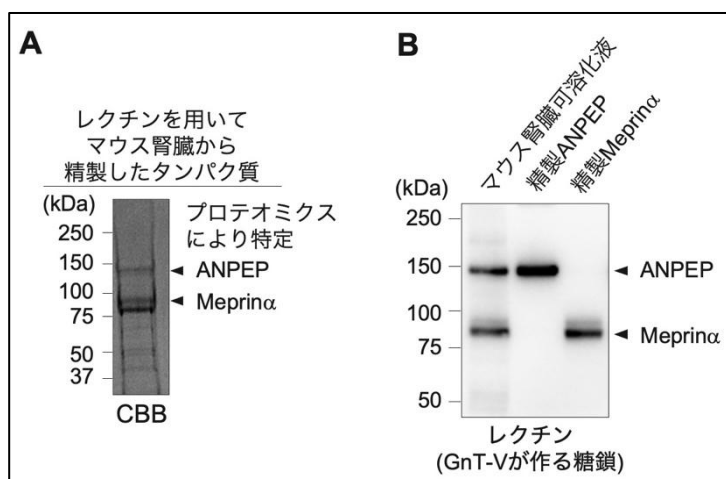
図2 A : GnT-V が作る枝分かれした糖鎖と特異的に結合するレクチンを用いて、この糖鎖を持つタンパク質をマウスの腎臓から精製し、矢頭で示されたタンパク質をプロテオミクスという手法で特定した。CBB は全てのタンパク質を染色する色素。B : 特定された ANPEP と Meprin \alpha をマウスの腎臓可溶化液から精製した。精製したタンパク質はどちらもレクチンと反応した。左のレーン、腎臓の可溶化液(タンパク質混合液)のサンプルを分析した。
