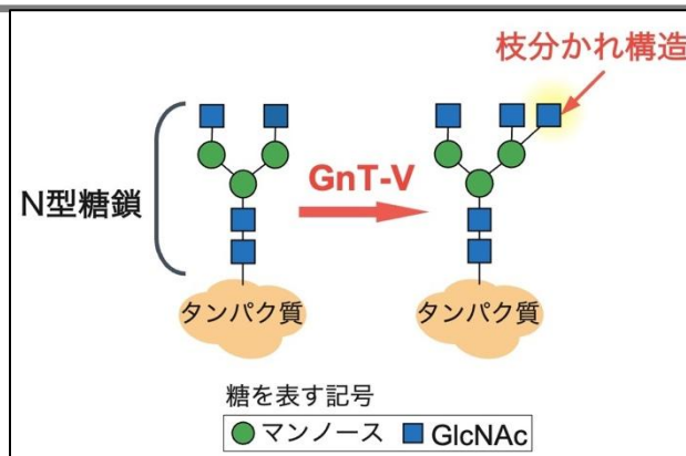
図1 GnT-V が作る糖鎖構造
