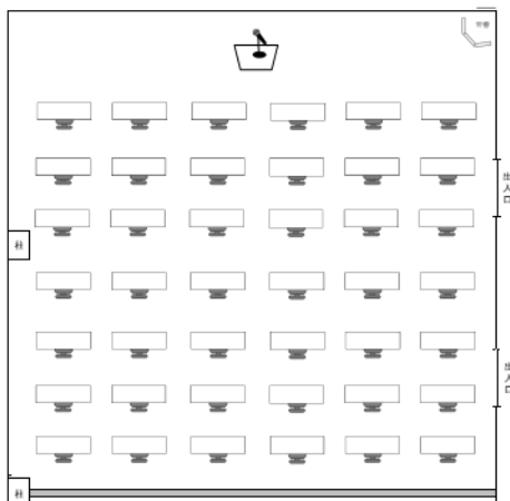
3 密回避レイアウト例 (185㎡・42 席)
