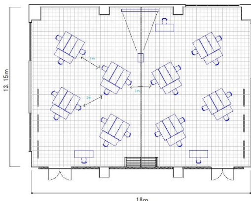
3 密回避 アイランドスタイル（島型）24 名の例 大会議室 A 236 m 2
