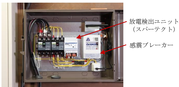
設置例
