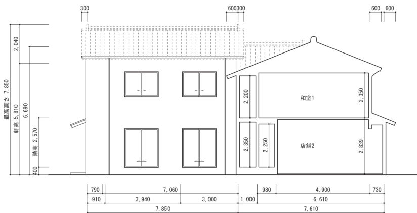
改修後 断面図 S=1/100
