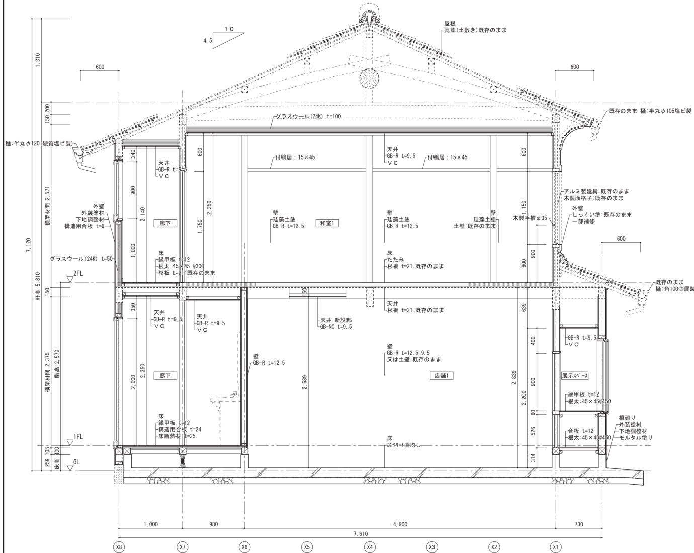
改修後 断面詳細図 1 S=1/30
