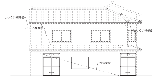
改修後 南東立面図 S=1/100
