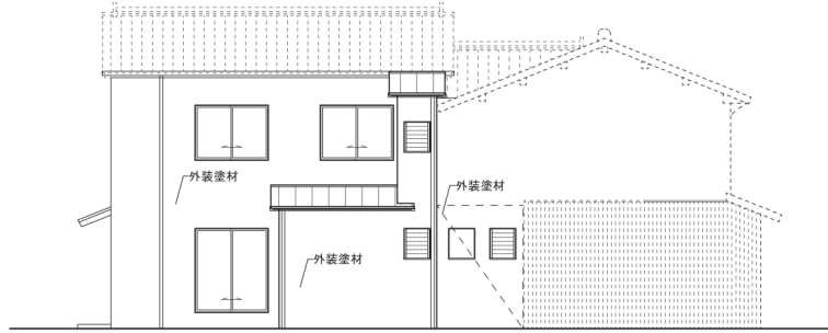
改修後 南西立面図 S=1/100
