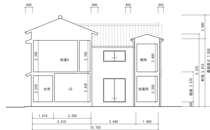
改修後 断面図 S=1/100
