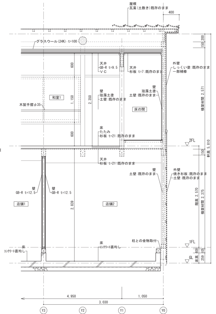
改修後 断面詳細図 2 S=1/30
