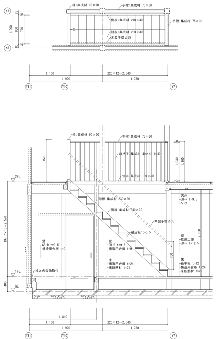
階段 詳細図 S=1/30
