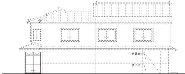
改修後 北東立面図 S=1/100
