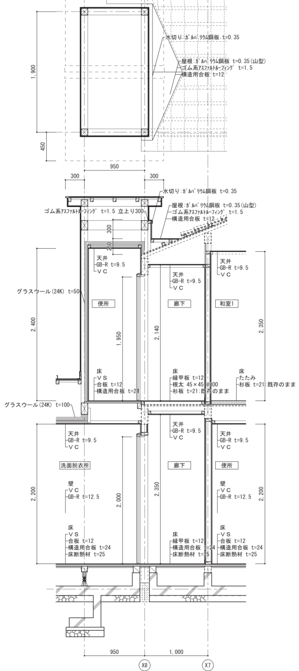
増築部 断面詳細図 S=1/30
