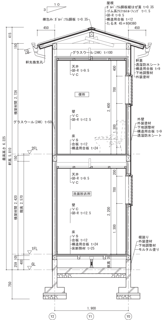
増築部 断面詳細図 S=1/30
