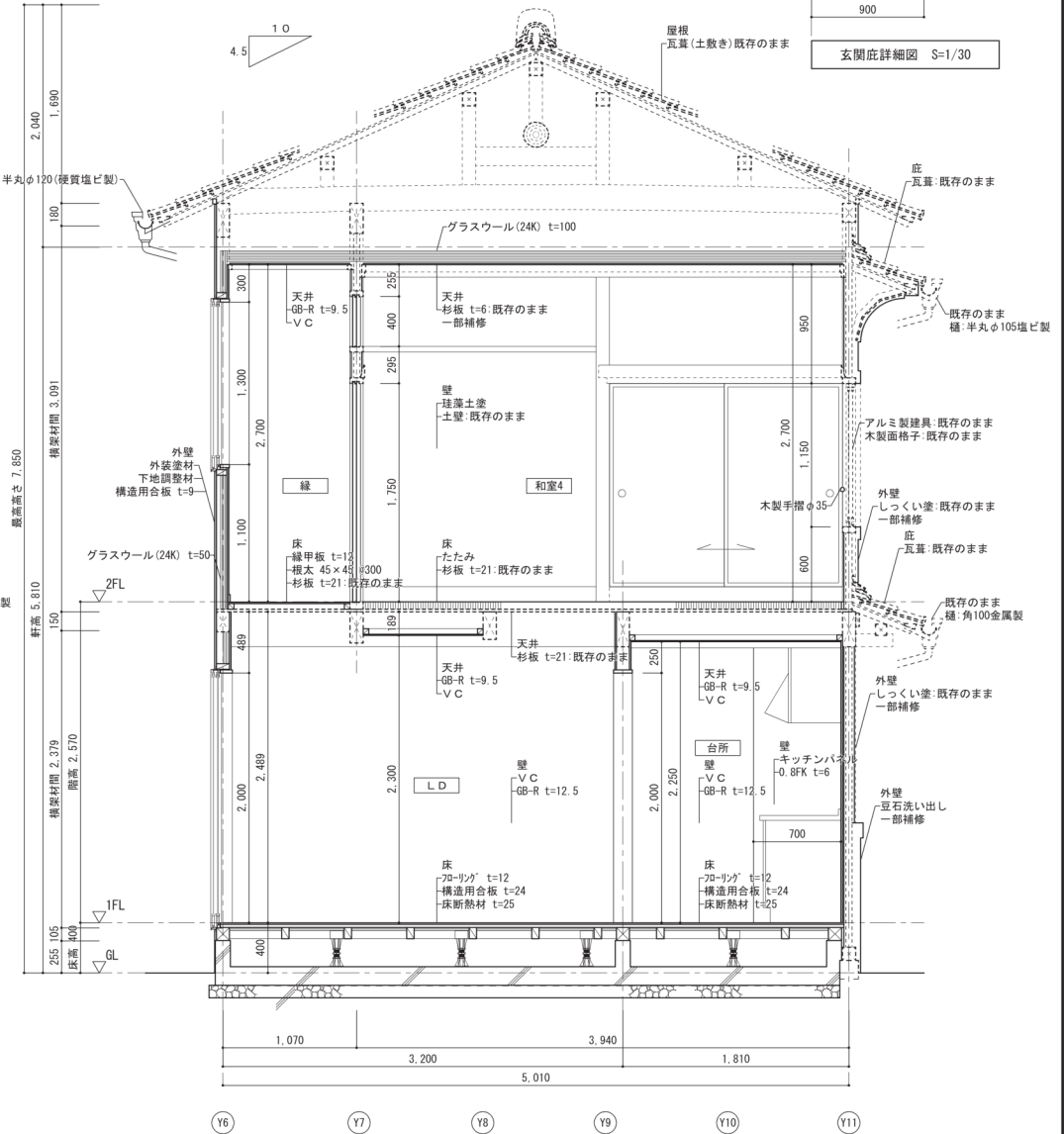
改修後 断面詳細図 3 S=1/30
