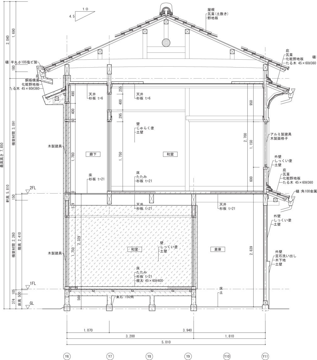
改修前 断面詳細図 3 S=1/30
