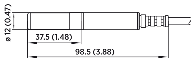
寸法(mm)
