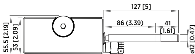
寸法(mm)
