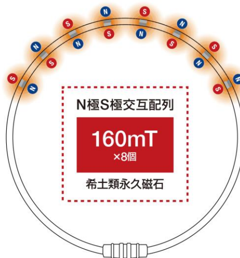
磁石配置図
