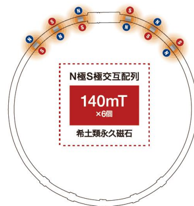
磁石配置図
