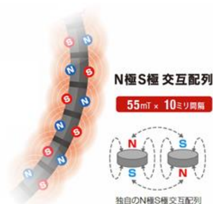
磁石配置 イメージ図
