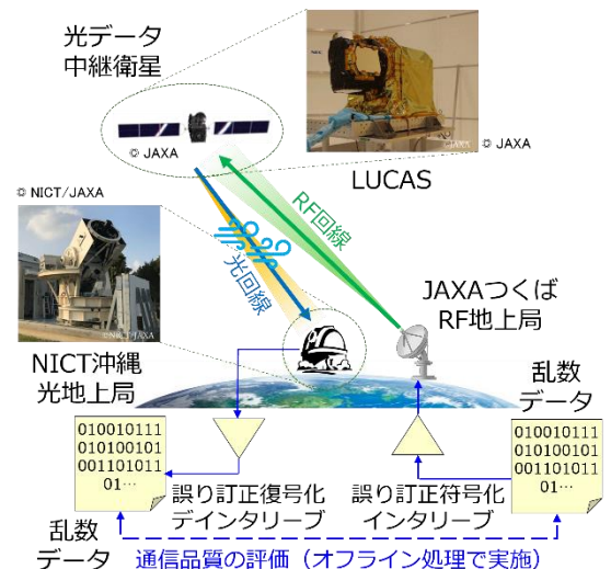
図1 次世代誤り訂正符号伝送実験のセットアップ
