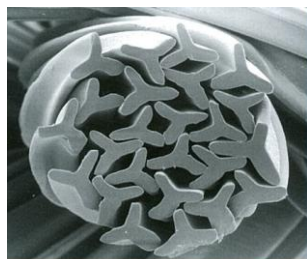
Y型断面ポリエステル糸「ソアリオン®Y」
