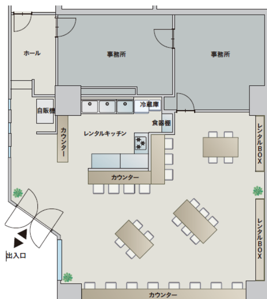
【配置図】
